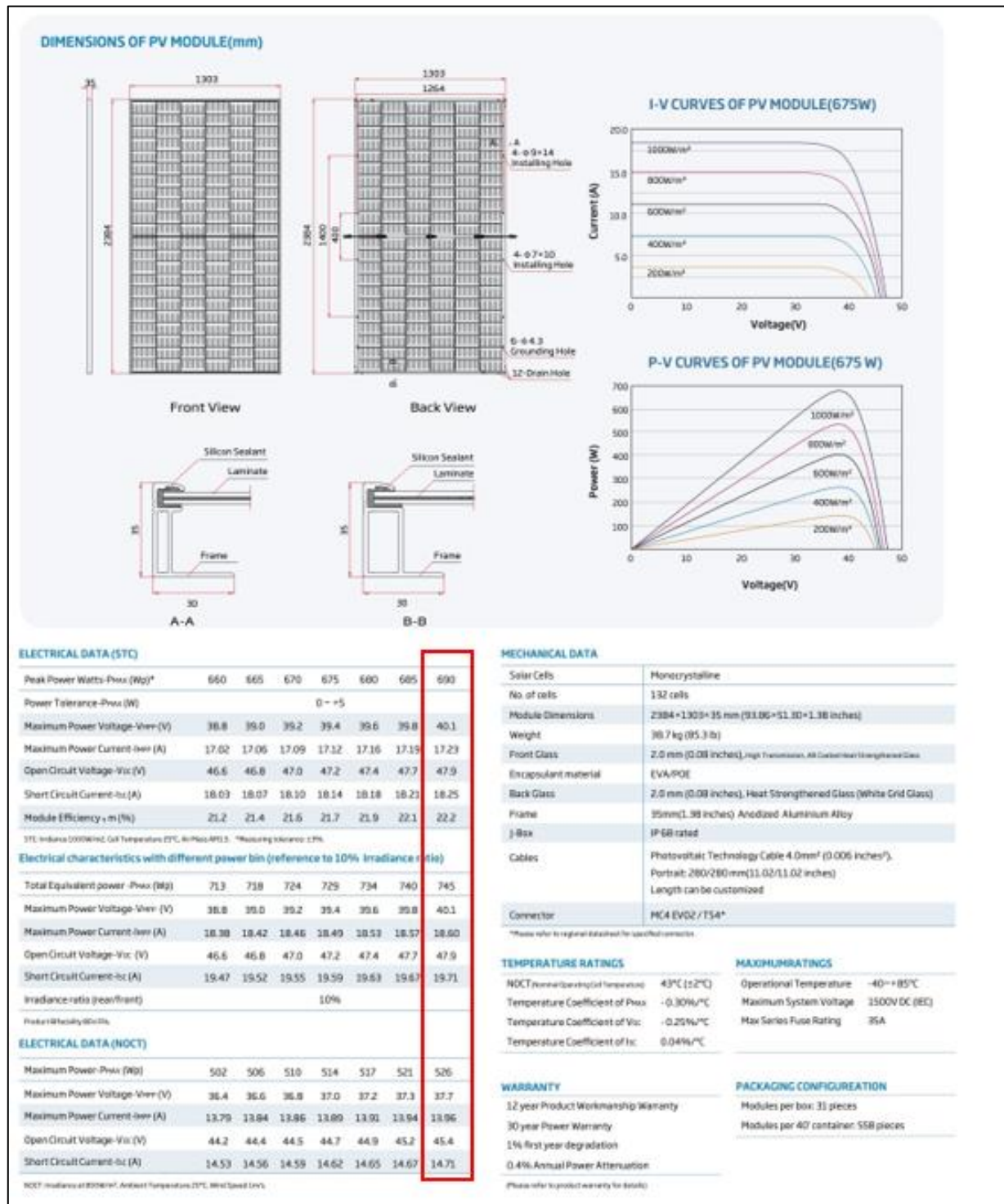
Εικόνα 5.3. Τεχνικά χαρακτηριστικά ΦΒ Πλαισίου TRINA BIF 690W
