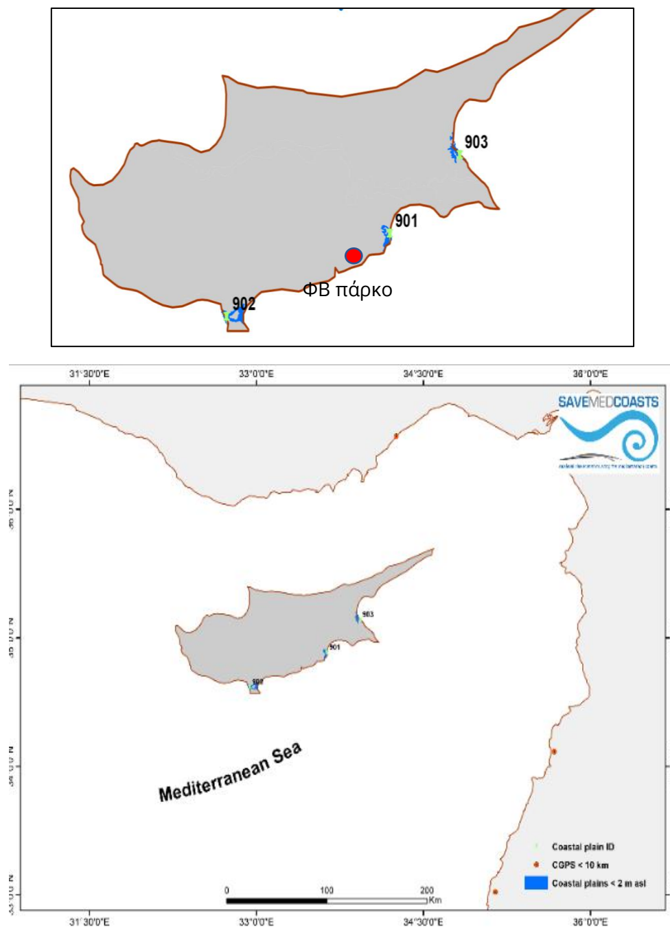
Εικόνα 7.25. Περιοχές υψηλού κινδύνου εξαιτίας της ανόδου της στάθμης της θάλασσας
